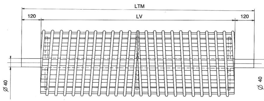
TYPE "TBSI" à spires inversées
