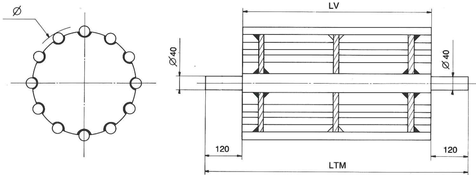
TYPE "TBCE" à cage d'écureuil
